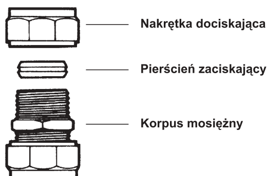
Rys. 2.6 Konstrukcja łącznika zaciskowego
