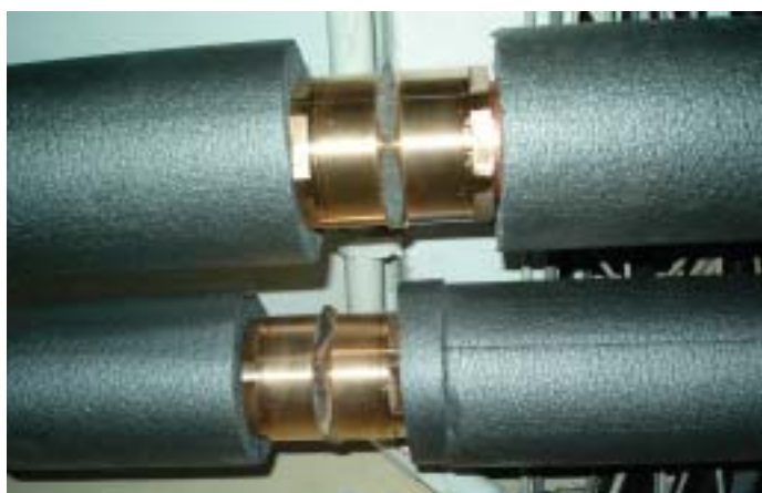
Rys.2.11 Kompensator typu O-yster Ø54
