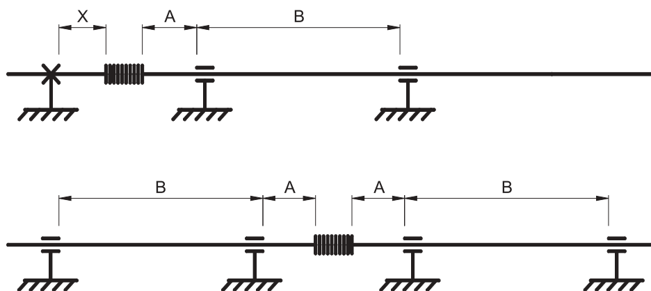
Rys. 3.15. Zasada rozmieszczania kompensatorów osiowych A = 4D ; B = 14D ; X = (0,5 \div 1,0)A
