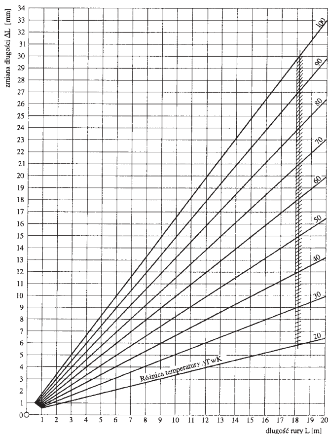
Rys. 3.5. Wydłużenie cieplne rur miedzianych
