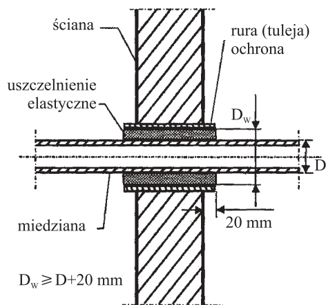
Rys. 3.2. Przykład przejścia przewodu przez strop
