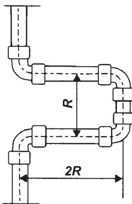
Rys. 3.10. Konstrukcja kompensatora z 4 kolan 90°
