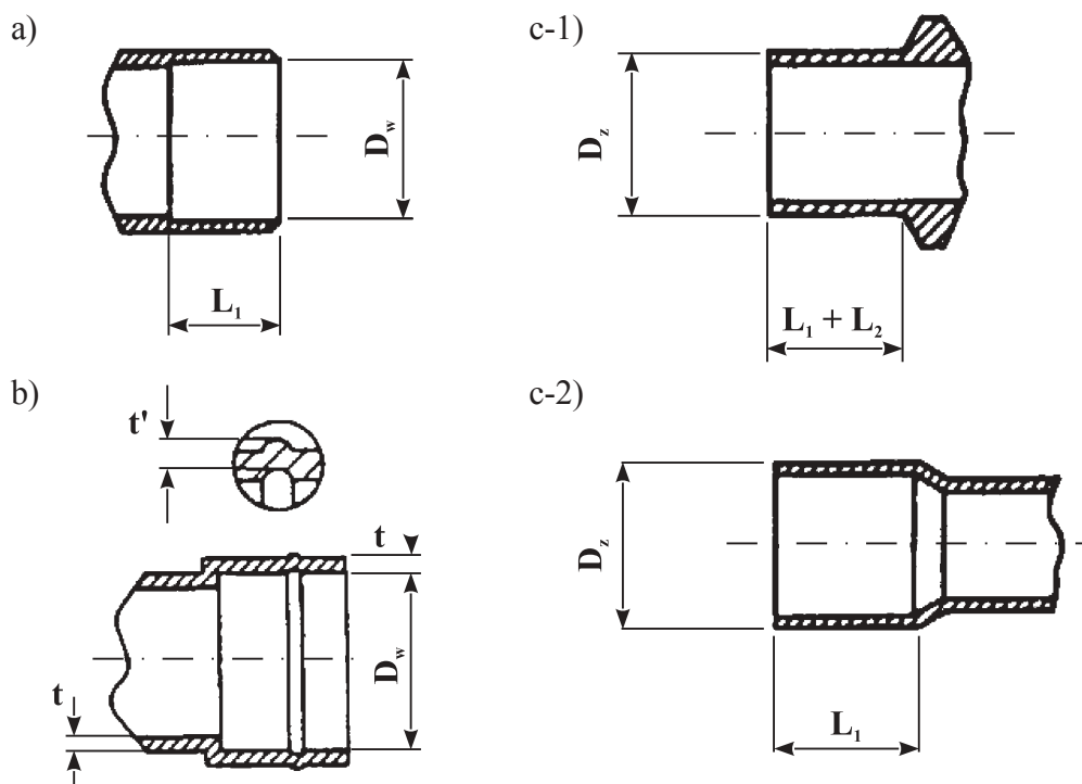
Rys. 2.5 Łączniki do lutowania kapilarnego (wymiary)
