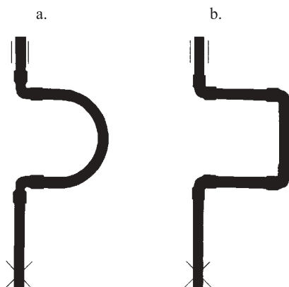
Rys. 3.9. Kompensatory U-kształtowe
