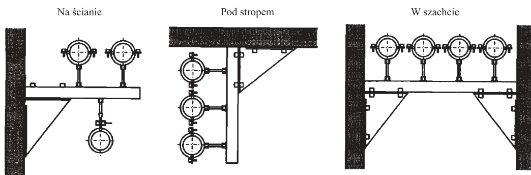
Rys.3.19. Sposób mocowania przewodów na wspornikach
