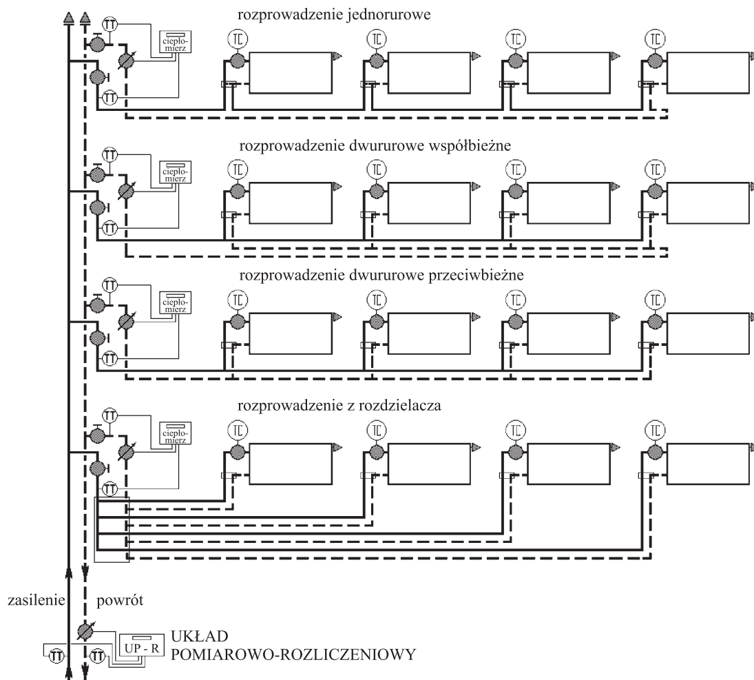
Rys. 5.1. Schematy mieszkaniowych rozprawadzeń instalacji c.o., w budynku wielorodzinnym
