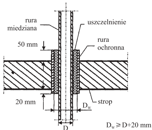
Rys. 3.1. Przykład przejścia przewodu przez ścianę
