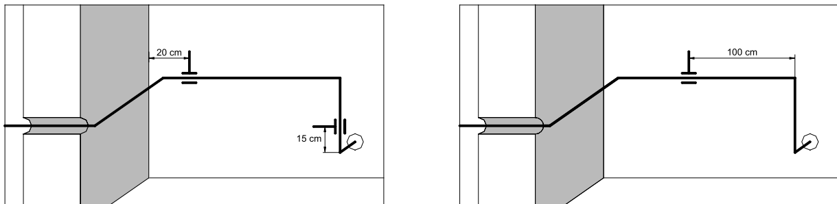
Rys.3.6. Przykład prowadzenia przewodu z zachowaniem kompensacji naturalnej
