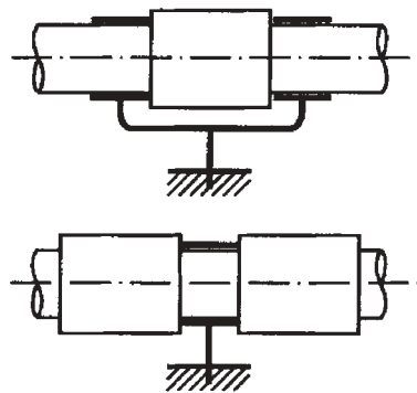
Rys. 3.16 Schematy budowy punktu stałego
