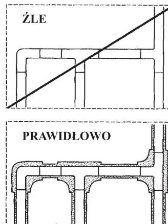
Rys. 3.7. Przykład układania przewodu miedzianego w bruzdzie pod tynkiem
