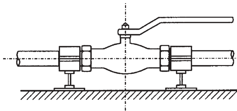
Rys. 3.17. Sposób mocowania armatury
