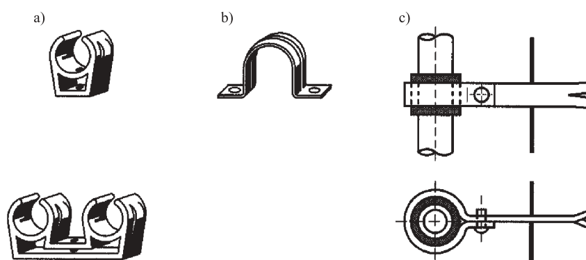
Rys. 3.18. Przykłady uchwytów do mocowania przewodów miedzianych
